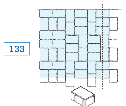
20,1x13,4 x 6 - environ 38 pièces/m 2
