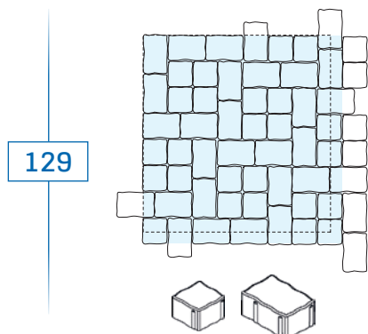
20,1x13,4 x 6 - environ 23 pièces/m 2 13,4 x 13,4 x 6 - environ 23 pièces/m 2
