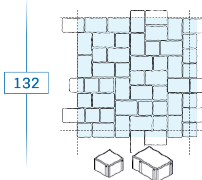
20,1x13,4 x 6 - environ 25 pièces/m 2 13,4 x 13,4 x 6 - environ 19 pièces/m 2
