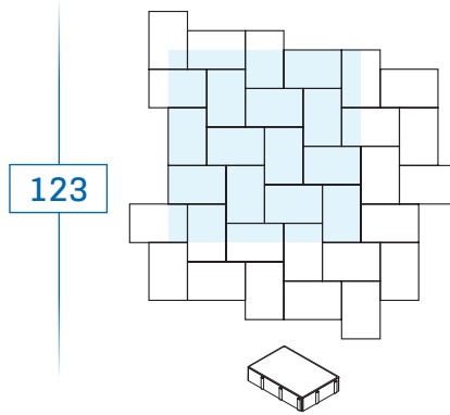
30 x 20 x 8 - environ 16,5 pces/m 2
