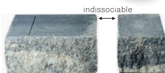
Élément de base 34 x 25 cm Poids / pce : 29,4 kg
