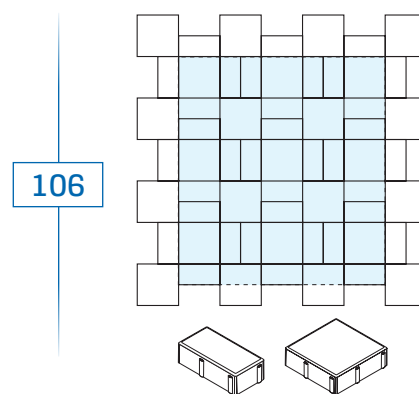
10 x 20 x 6 / 8 - environ 24 pces/m 2 20 x 20 x 6 / 8 - environ 13 pces/m 2
