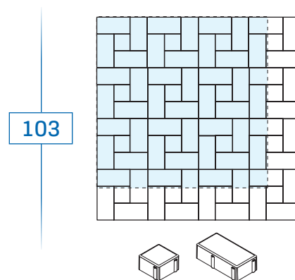
10 x 10 x 6 / 8 - environ 12 pièces/m 2 10 x 20 x 6 / 8 - environ 44,5 pièces/m 2
