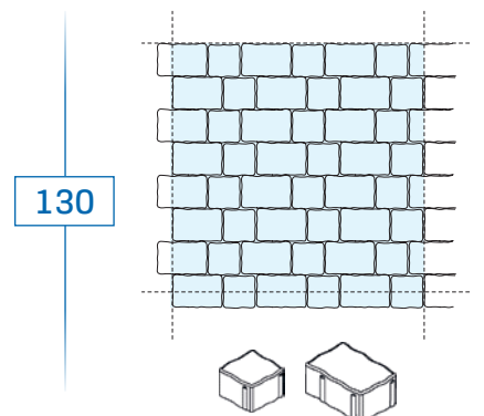
20,1x13,4 x 6 - environ 23 pièces/m 2 13,4 x 13,4 x 6 - environ 23 pièces/m 2
