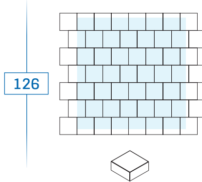
15 x 15 x 6 - environ 44,5 pces/m 2
