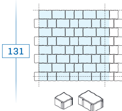
20,1x13,4 x 6 - environ 28 pièces/m 2 13,4x13,4 x 6 - environ 16 pièces/m 2
