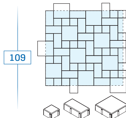
10 x 10 x 6 / 8 - environ 27 pièces/m 2 10 x 20 x 6 / 8 - environ 18,5 pièces/m 2 20 x 20 x 6 / 8 - environ 9 pièces/m 2
