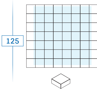
15 x 15 x 6 - environ 44,5 pces/m 2
