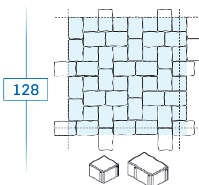
20,1x13,4 x 6 - environ 28 pièces/m 2 13,4x13,4 x 6 - environ 14 pièces/m 2
